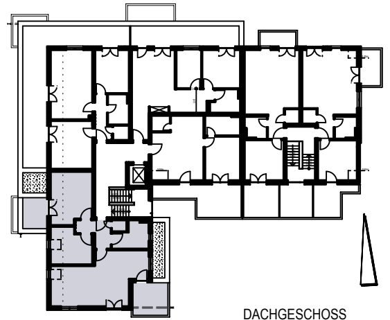
DACHGESCHOSS
